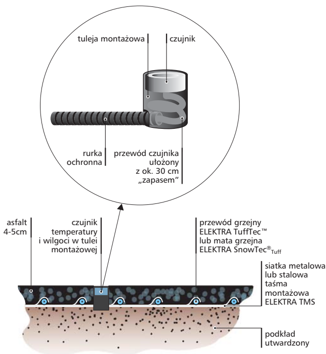
Przykład instalacji czujnika ETOG-56T w nawierzchni asfaltowej
